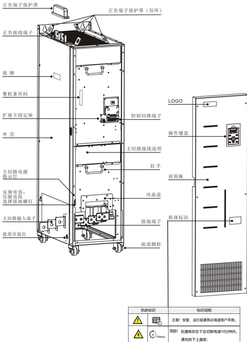
图 1-3 产品部件示意图【LS300T200G/220P-C ~ LS300T630G/710P-C】
