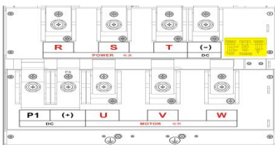
图 3-11 LS300T132G/160P ~ L300T450G/500P 主回路端子分布图
