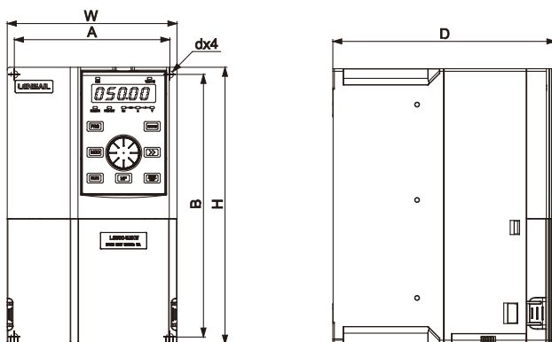
图 1-4 LS300T0.7GB/1.5PB ~ LS300T18.5GB/22PB, LS300-2T0.7GB/1.5PB ~ LS300-2T7.5GB/11PB 外型尺寸及安装尺寸示意图
