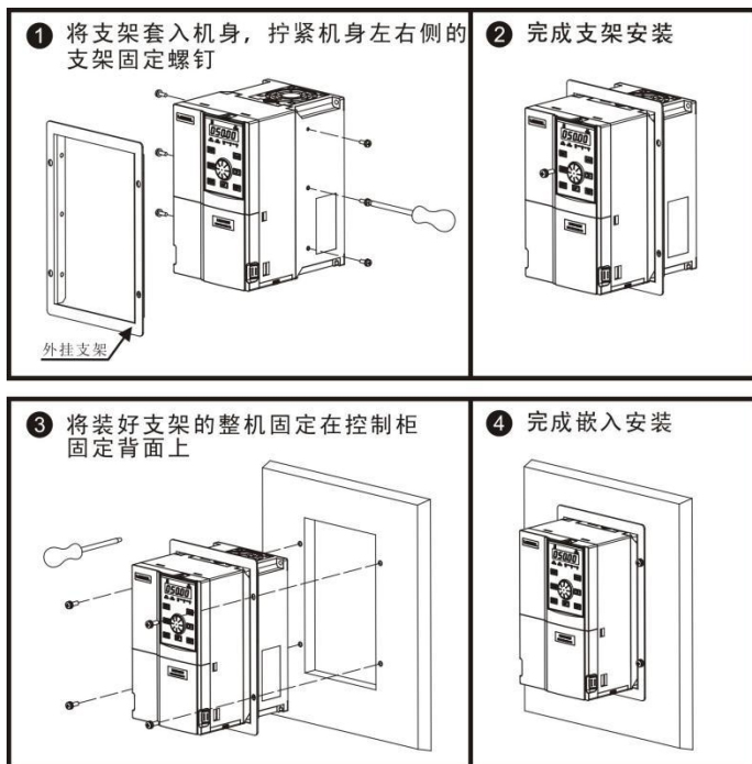
图 3-4 LS300T0.7GB/1.5PB ~ LS300T18.5GB/22PB, LS300-2T0.7GB/1.5PB ~ LS300-2T7.5GB/11PB 机型嵌入式安装示意图
