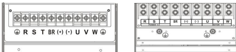
图 3-10 LS300T22GB/30PB ~ LS300T110G/132P, LS300-2T11GB/15PB ~ LS300-2T55G/75P 主回路端子分布图
