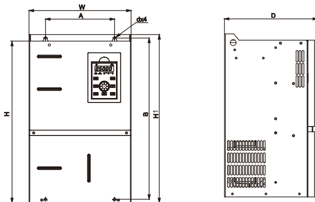
图 1-5 LS300T22GB/30PB~LS300T160G/200P, LS300-2T11GB/15PB~LS300-2T55G/75P 外型尺寸及安装尺寸示意图
