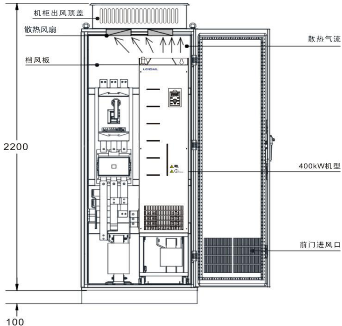
图 3-7 顶部风扇抽风机柜示意图 (机柜顶部带抽风风扇)
