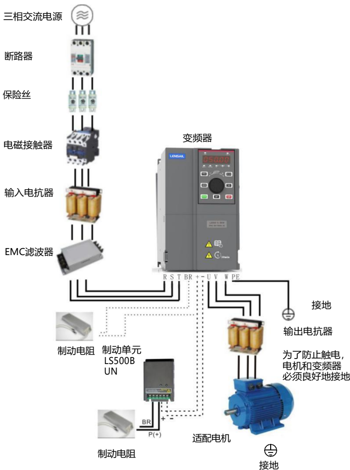
图 2-1 LS300 系列系统构成
