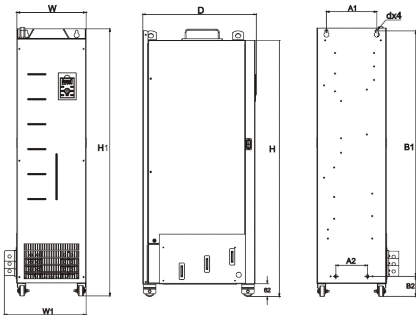
图 1-7 LS300T200G/220P-C ~ LS300T630G/710P-C 外型尺寸及安装尺寸示意图
