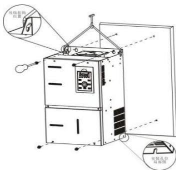
图 3-3 LS300T22GB/30PB ~ LS300T450G/500P, LS300-2T11GB/15PB ~ LS300-2T55G/75P 机型壁挂式安装示意图
