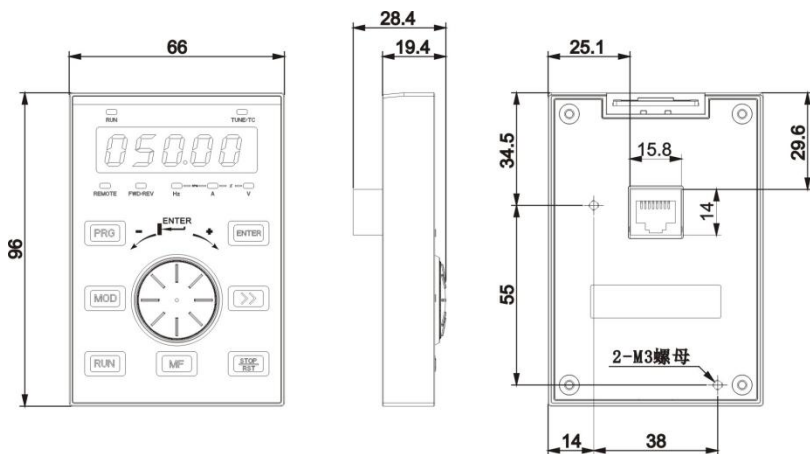
图 2-2 LS500LEDK 键盘尺寸 (单位: mm)
